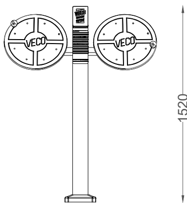
ALÇADO FRONTAL FRONT VIEW
