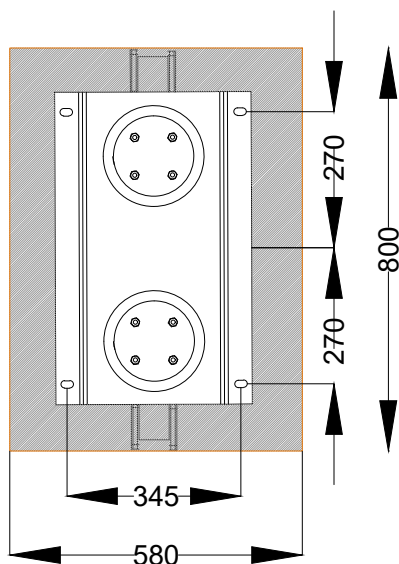
PLANTA . ESQUEMA DE FIXAÇÃO PLAN . INSTALLATION PLAN
