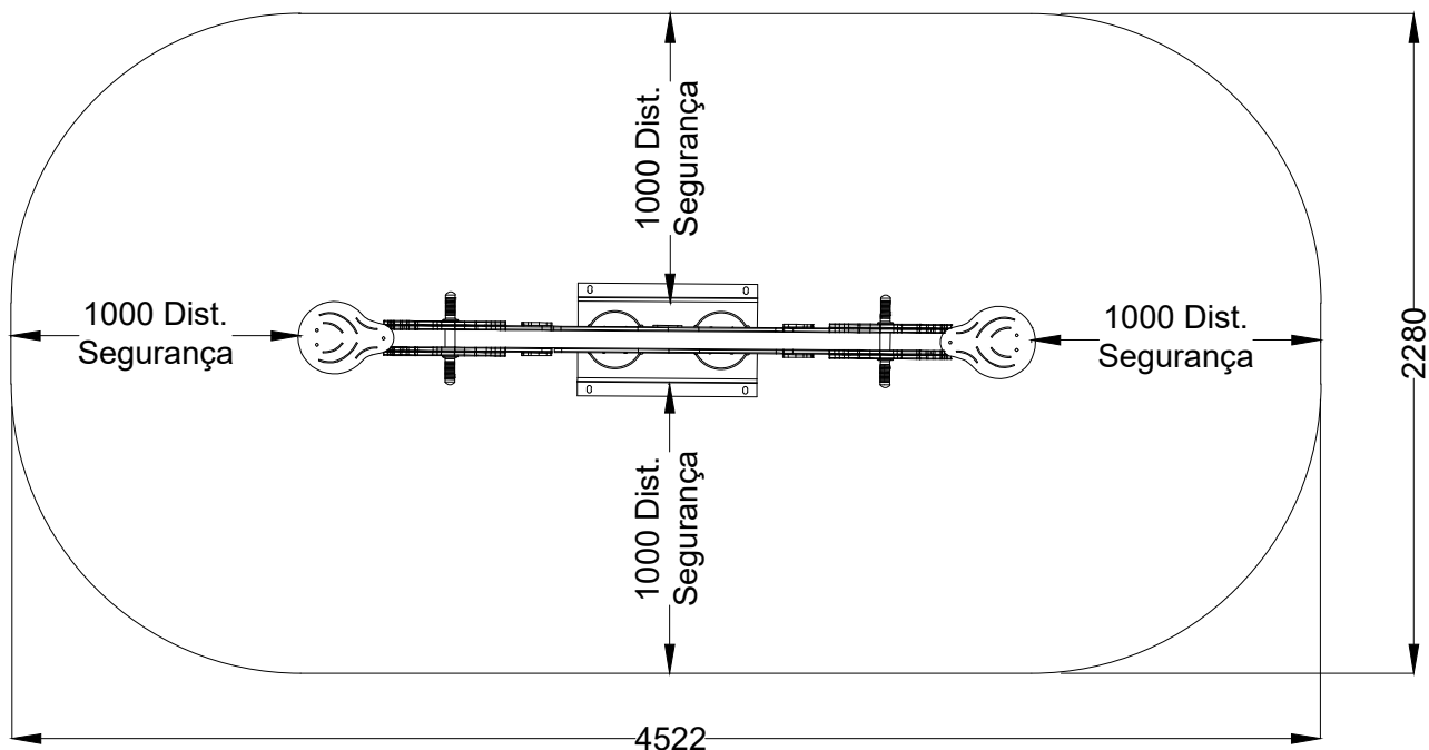
PLANTA - ESPAÇO DE SEGURANÇA NECESSÁRIO PLAN - SAFETY SPACE REQUIRED
