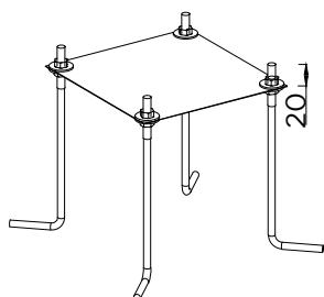
PLANTA . ESQUEMA DE FIXAÇÃO PLAN . INSTALLATION PLAN
