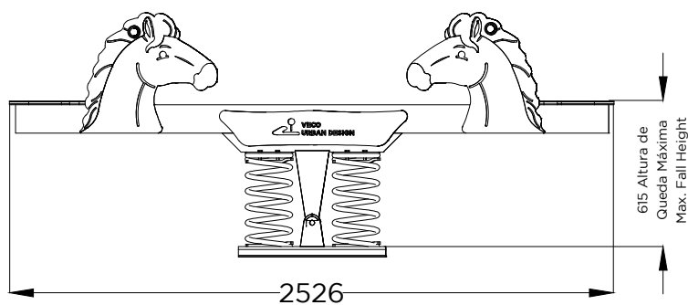
ALÇADO LATERAL SIDE VIEW
