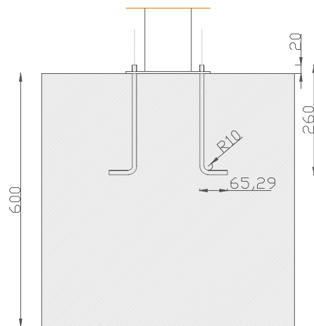
ALÇADO
