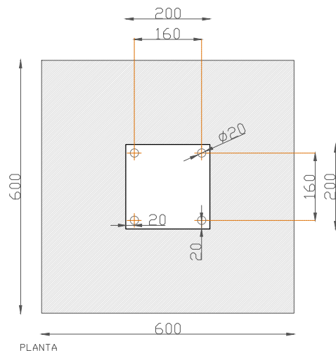
PLANTA
