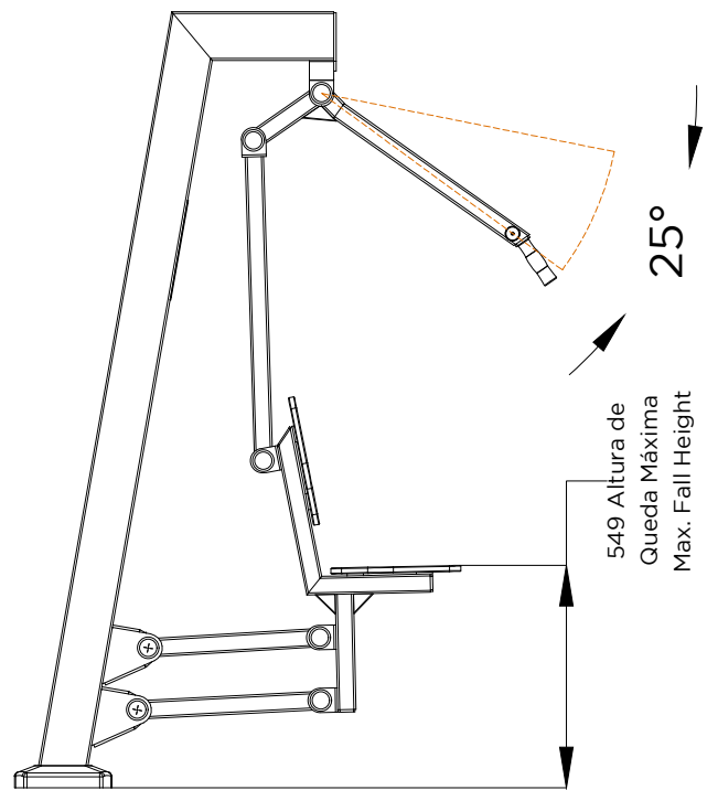
ALÇADO LATERAL SIDE VIEW
