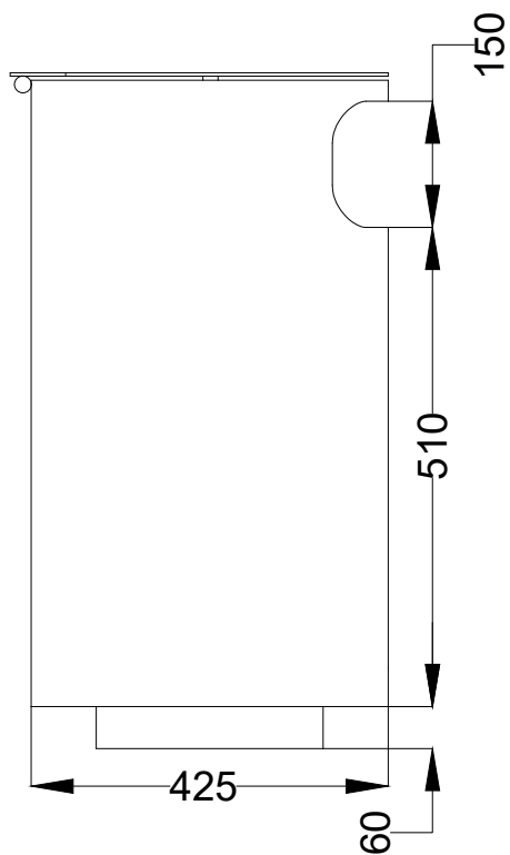
ALÇADO LATERAL SIDE VIEW
