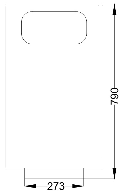
ALÇADO FRONTAL FRONT VIEW
